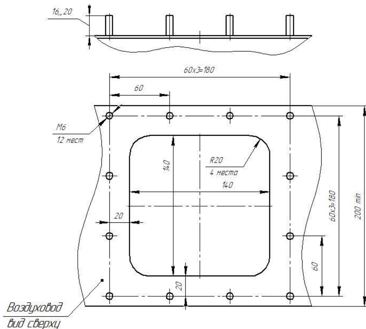
Рисунок 9 – Место для установки комплекта
