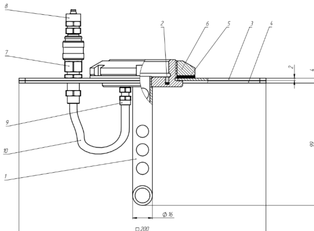
Рис. 10 Общий вид комплекта.
