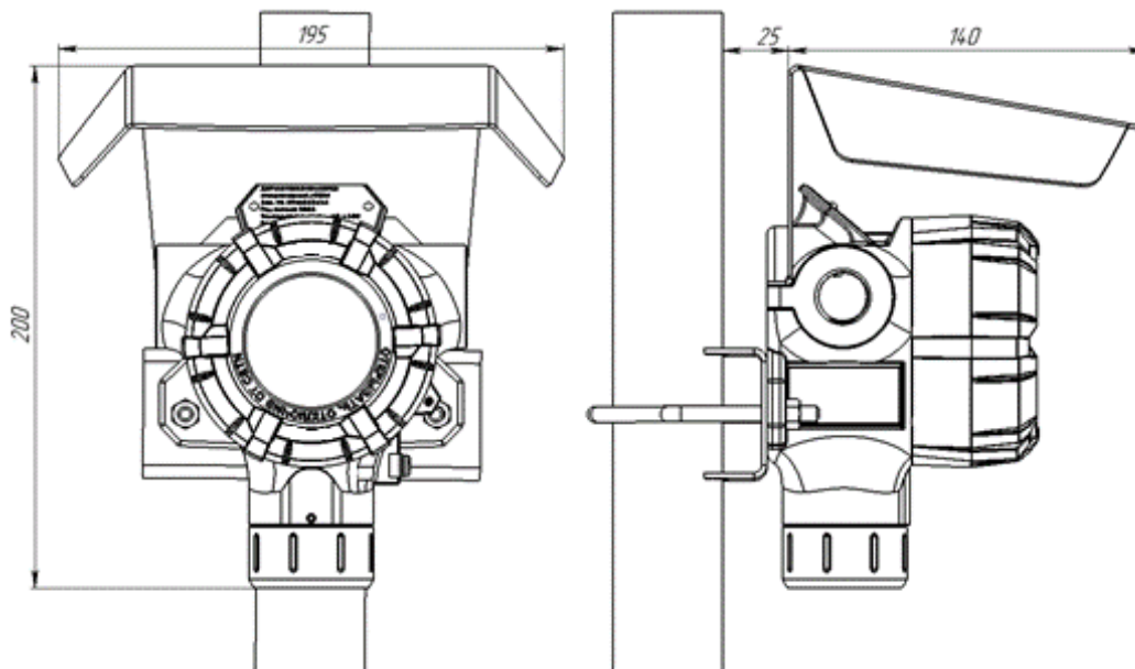
Рисунок 11- Монтаж козырька газоанализатора
